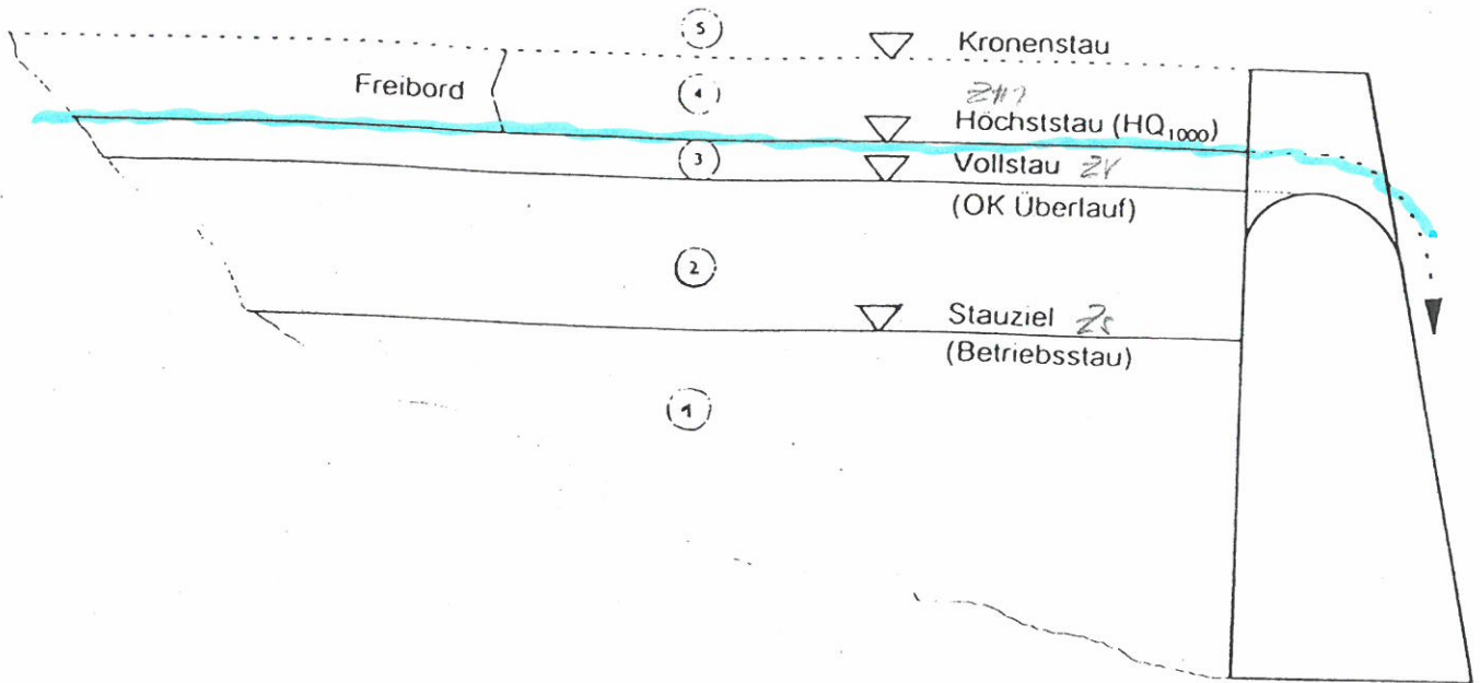
Längsschnitt Stauanlage
